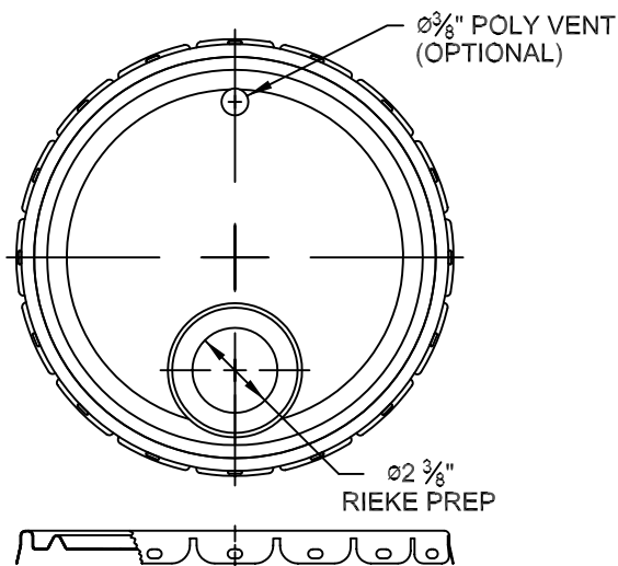
Rieke Prep:
